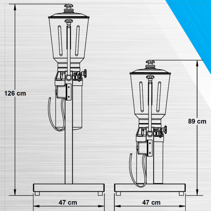
Vista lateral
